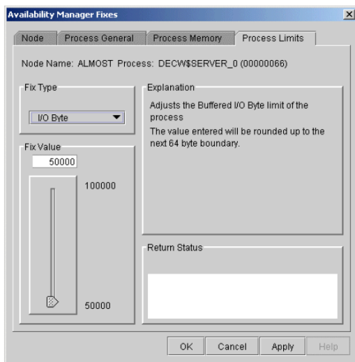
Figure 6.18. I/O Byte
